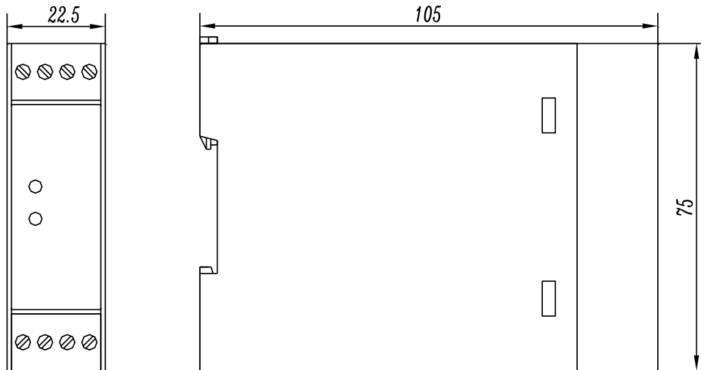
图 1.2 外形尺寸图
